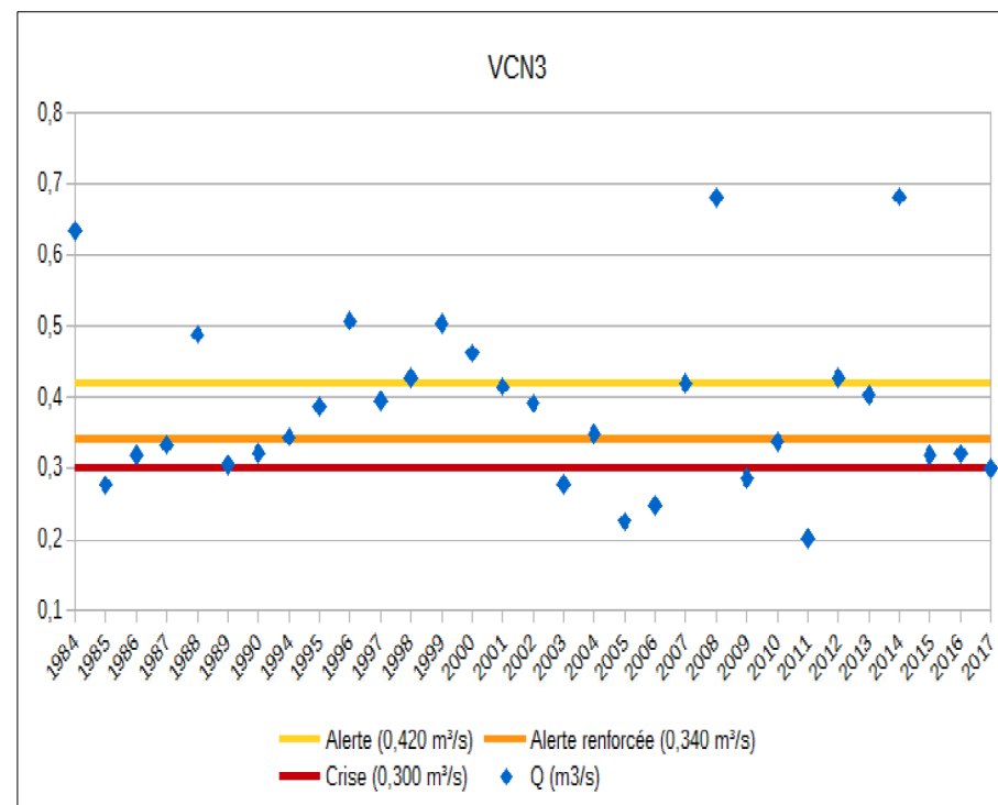
Station hydrométrique de Mende aval - graphique des plus bas débits de 1984 à 2017
