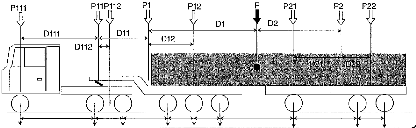
Ensemble routier : tracteur 2 ou 3 essieux avec semi-remorque et remorque de type boggie
